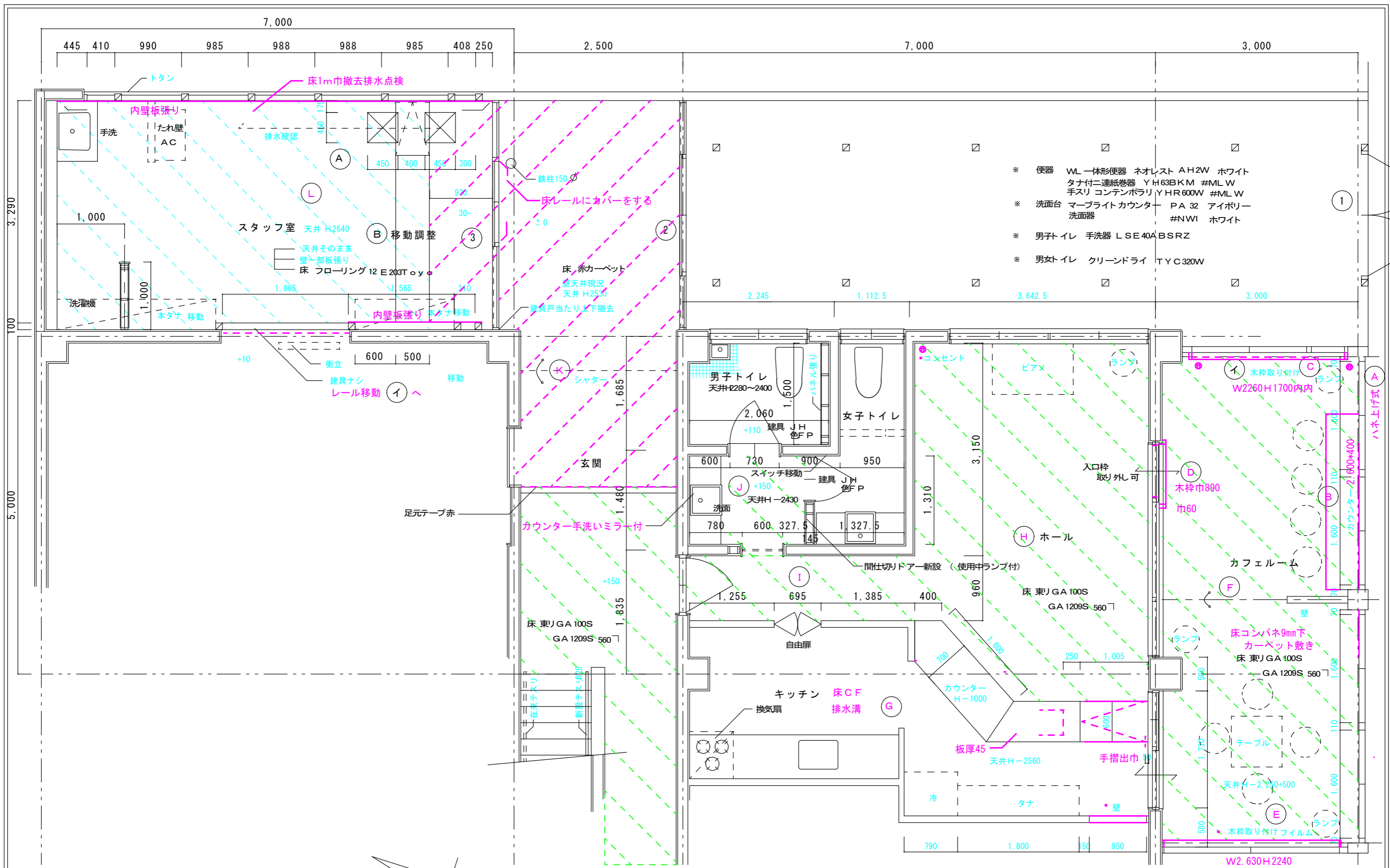
平面図 S=1/50
